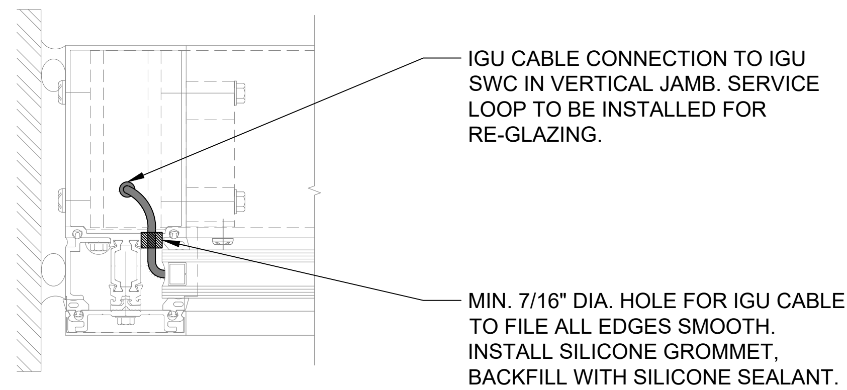
DETAIL 4 LEFT JAMB
